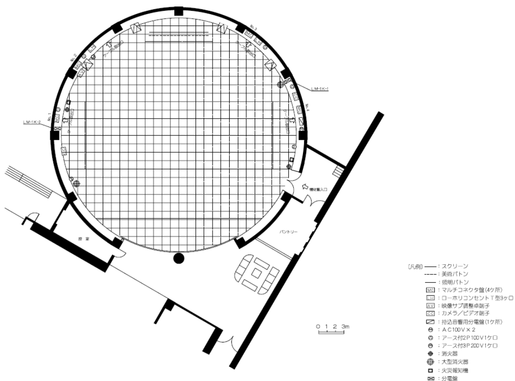
多目的ホール平面図
